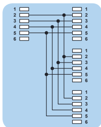
Adaptador RJ11 macho - 3x RJ11 hembra 6V/4Ctos.
