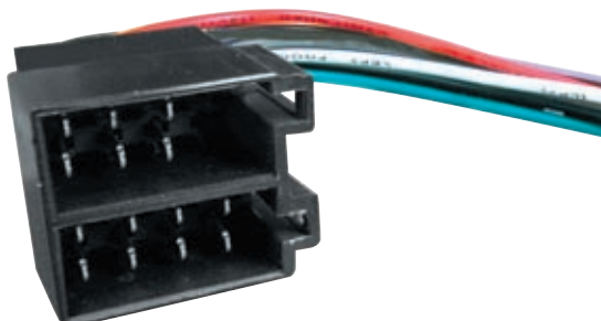
WIR021 Conector hembra. 6+8 conexiones / 16 vías.
